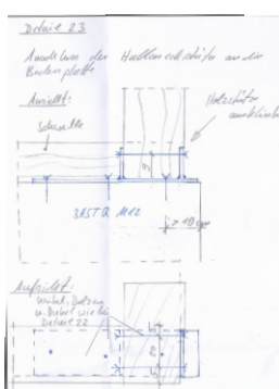
Holzkonstruktion, Details: Anschluss der Holzstützen an die Bodenplatte über Bolzen und Dübel
