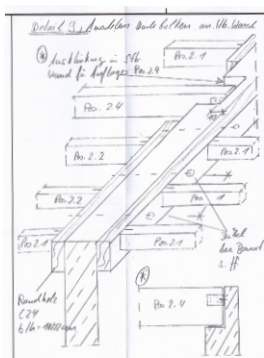
Holzkonstruktion, Details: Anschluss der Dachbalken an die Stahlbetonwand durch Scheibendübel
